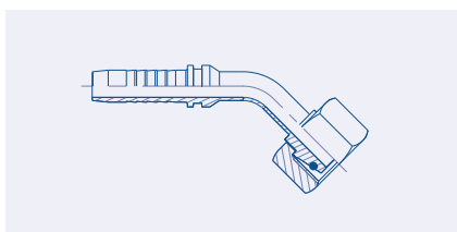
Hembra Métrica Giratoria Serie Ligera Asiento Cono 24°, Codo 45° (DKOL 45)
