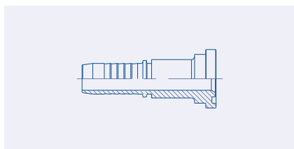
Flange SAE Recta (código 61) 3000 PSI (SFL)
