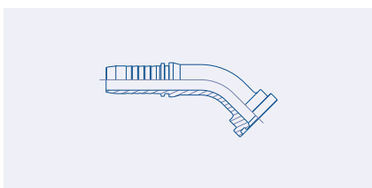
Flange SAE (código 61) 3000 PSI, Codo 45° (SFL 45°)
