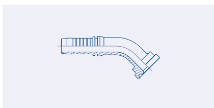
Flange SAE (código 62) 6000 PSI, Codo 45° (SFS 45°)
