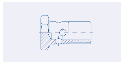
Perno Banjo Métrico
