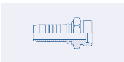
Macho Métrico Serie Ligera Asiento Cono 24° (CEL)
