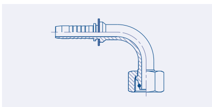
Hembra Métrica Giratoria Serie Ligera Asiento Cono 24°, Codo 90° (DKOL 90)
