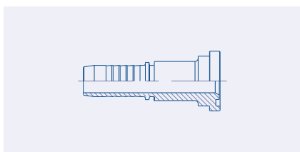
Flange SAE Recta (código 62) 6000 PSI (SFS)
