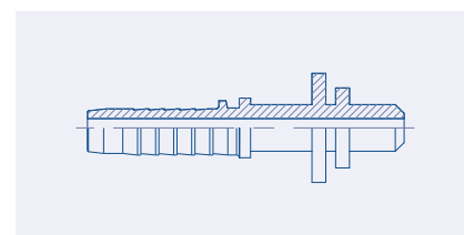
Espiga Hidrolavadora con O'ring (Karcher)
